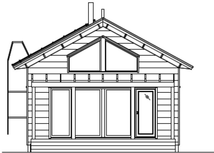
JULKISIVU 1
