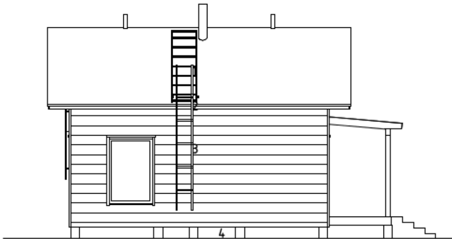
JULKISIVU 4
